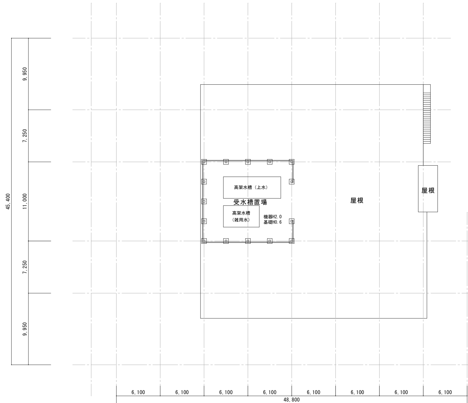
R階平面図
