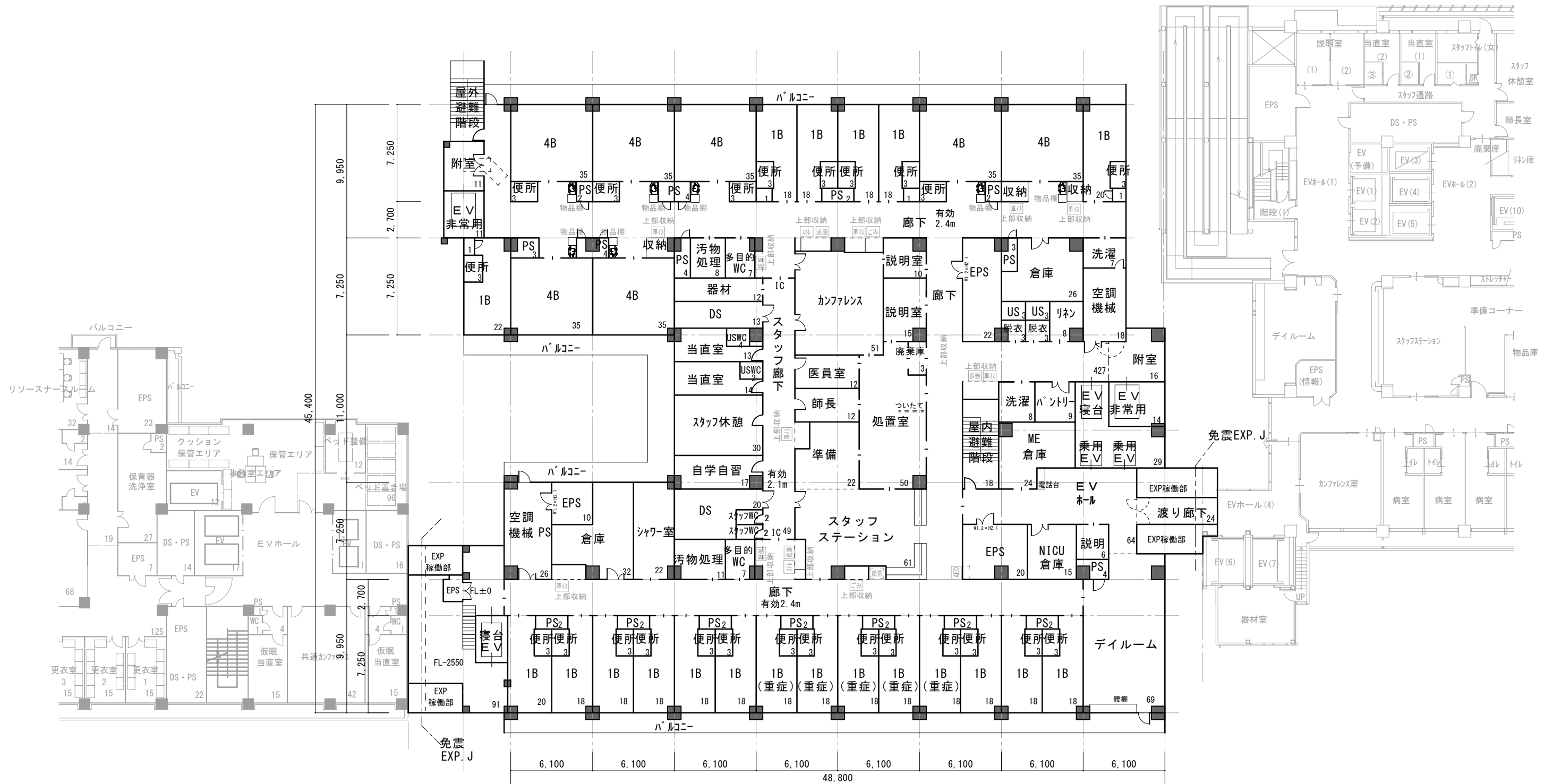
7階平面図
