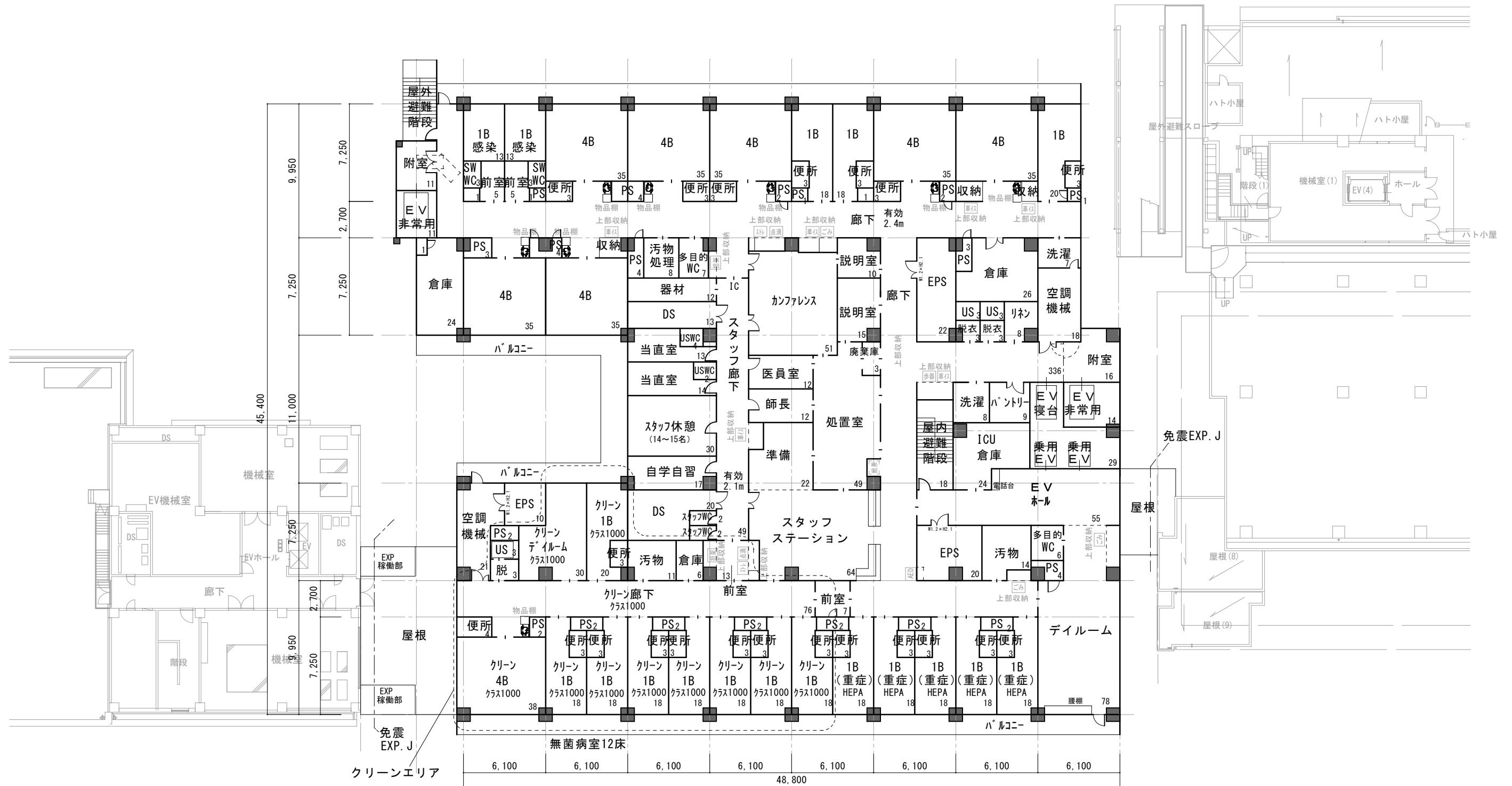
8階平面図
