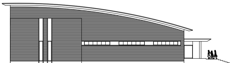
■ 東立面図 S=1/400 ■
