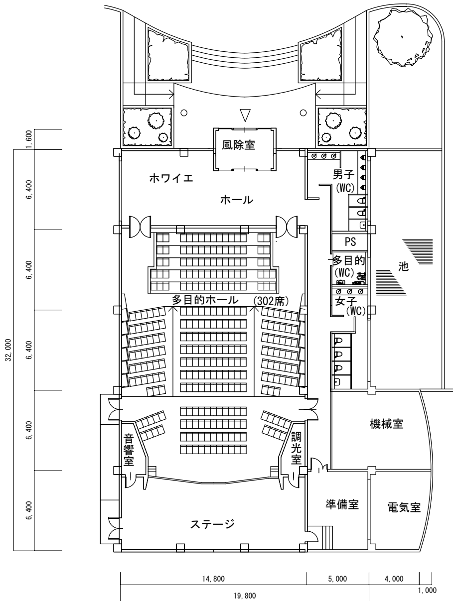
医学部会館（300席） S=1/300
