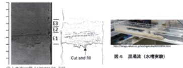
図3 左:写真、右:スケッチ。E1-E3(岩井 ほか, 2004)のタービダイトモデルの断面図。
