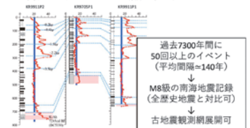
図4 土佐ばえ海盆(土佐湾)のタービダイト層の年代推定と南海トラフ地震(2004年)との関係を示す。
