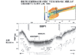
図2 土佐ばえ海盆の地下構造(南海トラフ)とコア試料採取地点(岩井 ほか, 2004)に示す。
